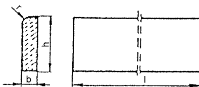
Rys. 1. Kształt betonowego obrzeża chodnikowego
