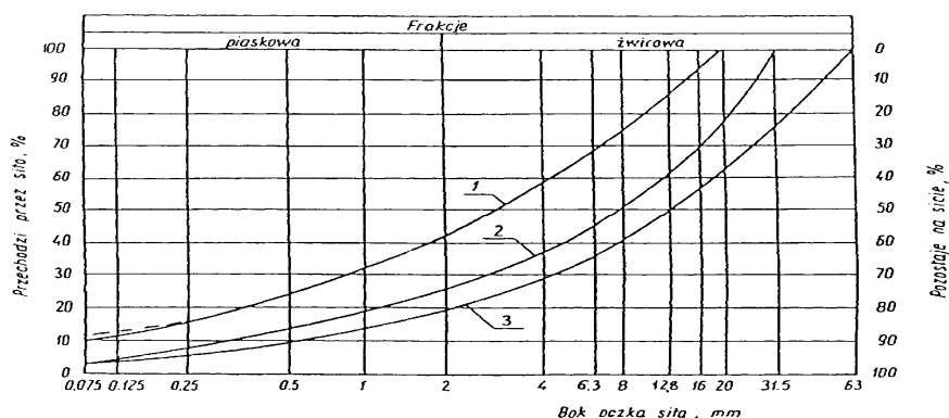
Rys.1. Pole dobrego uziarnienia kruszyw przeznaczonych na podbudowy wykonywane metodą stabilizacji mechanicznej.
