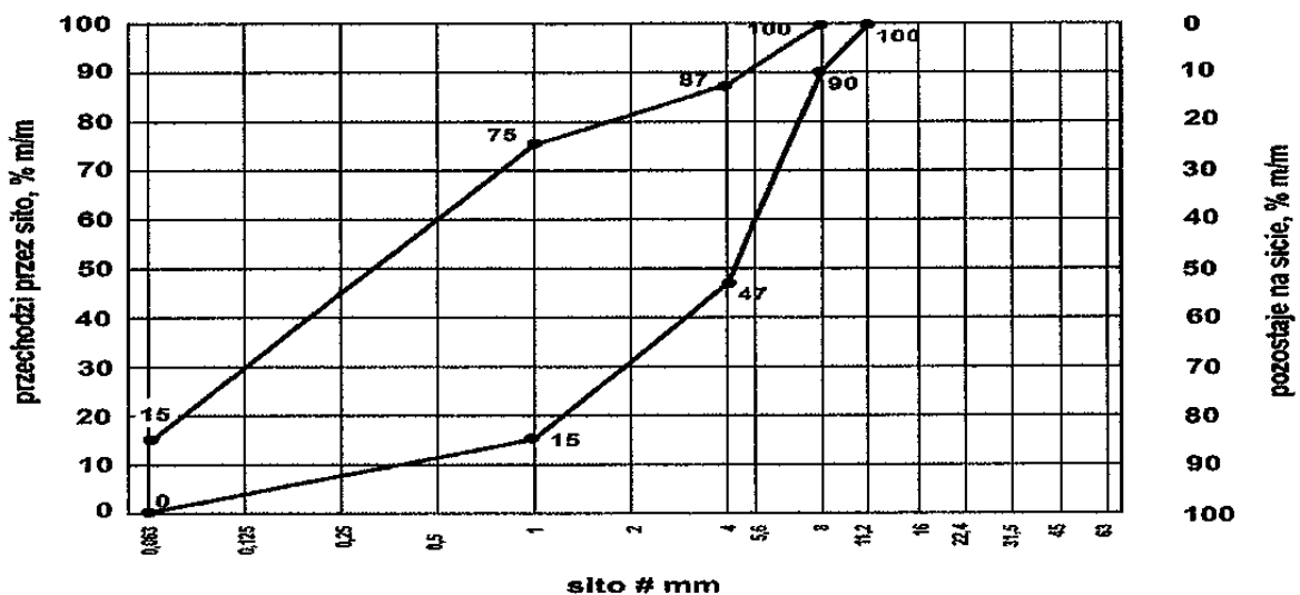
Rys. 1. Krzywe graniczne uziarnienia mieszanki kruszywa niezwiązanej 0/8 mm do nawierzchni
