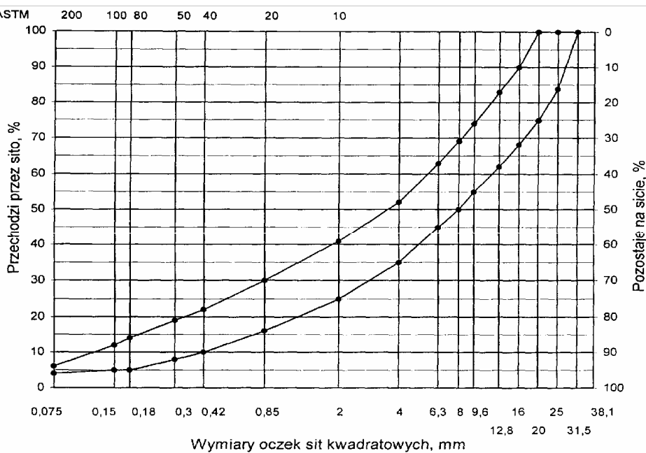
Rys. 11. Krzywe graniczne uziarnienia mieszanki mineralnej BA od 0 do 25 mm do warstwy wiążącej, wyrównawczej i wzmocniającej nawierzchni drogi o obciążeniu ruchem od KR3 do KR6
