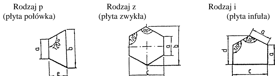
Rysunek 1. Kształt płyt betonowych
