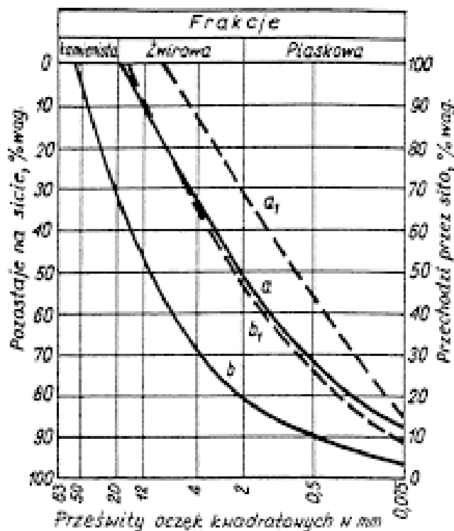
Rys.1. Obszar uziarnienia optymalnych mieszanek żwirowych
