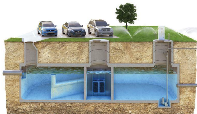
Ryc. 11 Zbiorniki podziemne, źródła (od lewej): https://www.uponor.pl ; https://ecol-unicon.com/produkty/produkty-deszczowe/zbiorniki-retencyjne-hydrozone/
